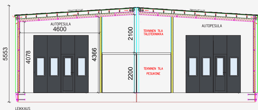
TUPLAHALLIN LEIKKAUSKUVA.
