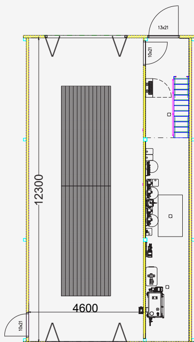
SINKKUHALLIN POHJA.
